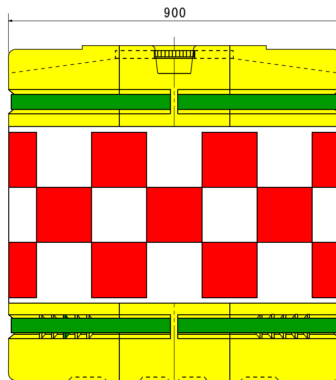
正面図 A 矢視
